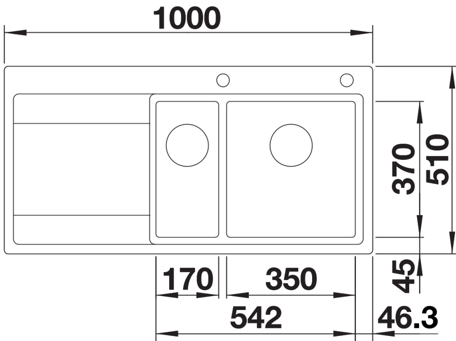
Bovenaanzicht
