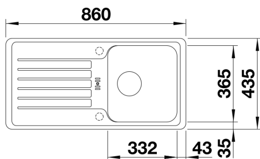
Bovenaanzicht
