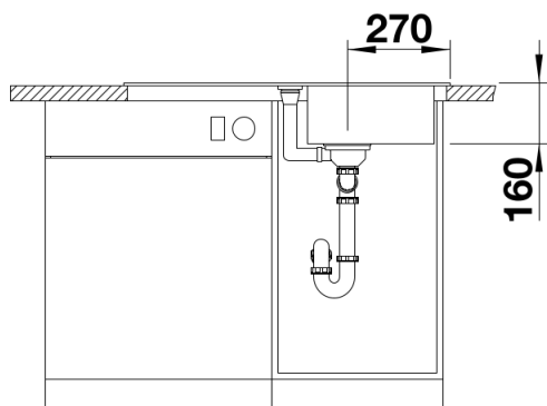
Vooraanzicht
