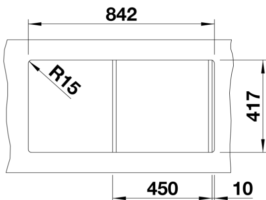
Uitgesneden
