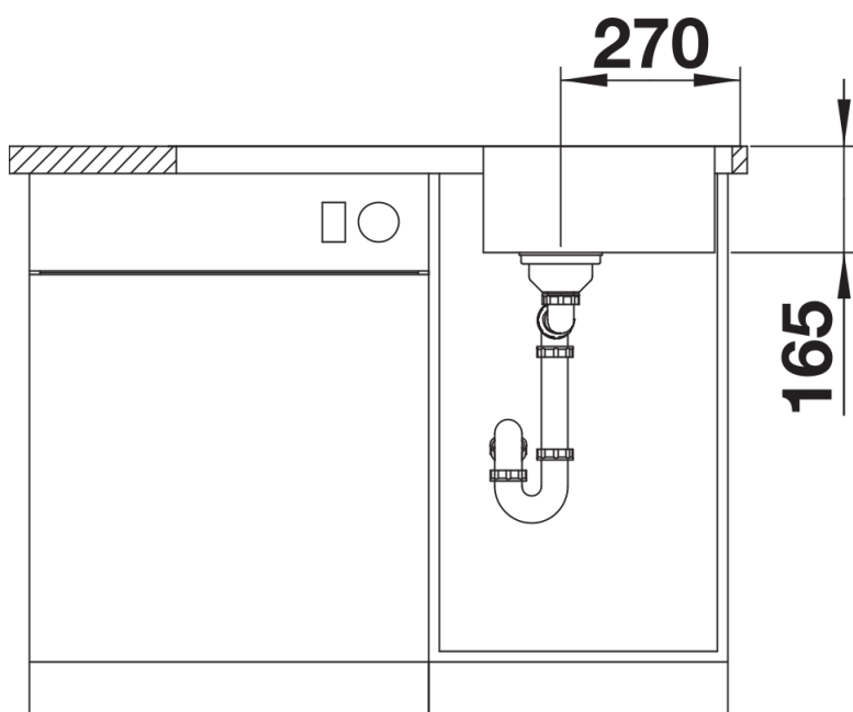
Vooraanzicht
