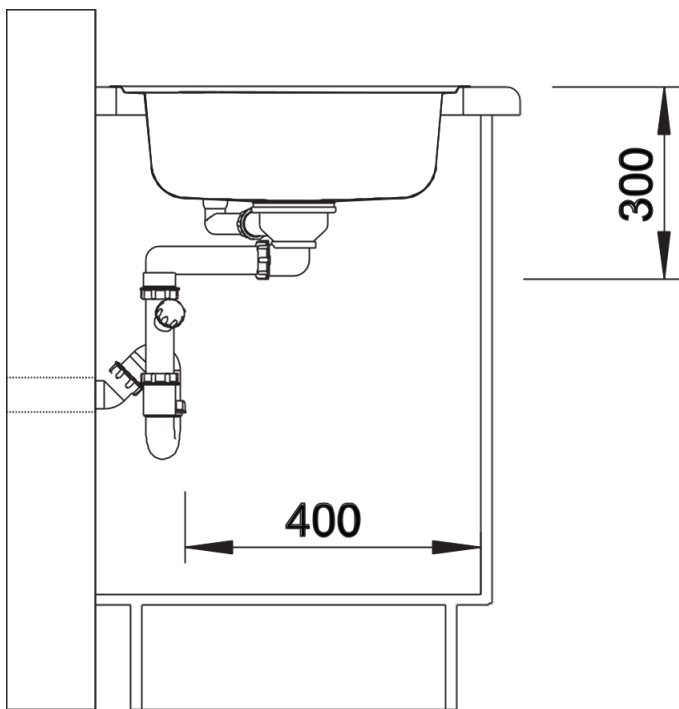
Zijaanzicht
