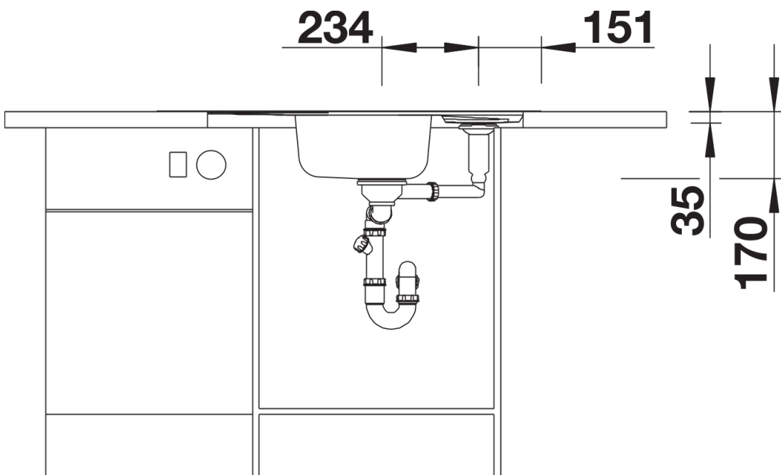
Vooraanzicht
