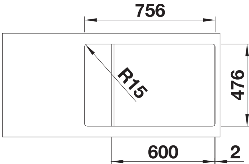
Uitgesneden
