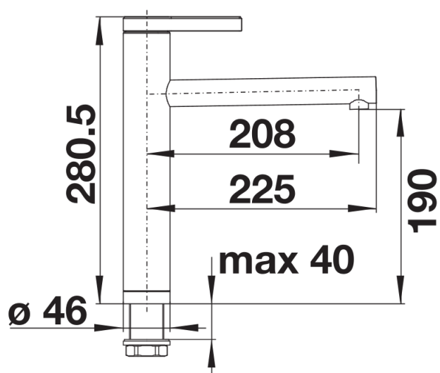
Zijaanzicht
