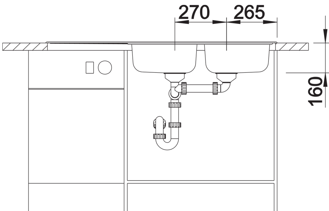
Vooraanzicht
