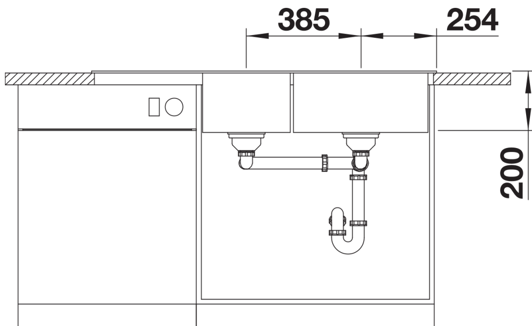
Vooraanzicht
