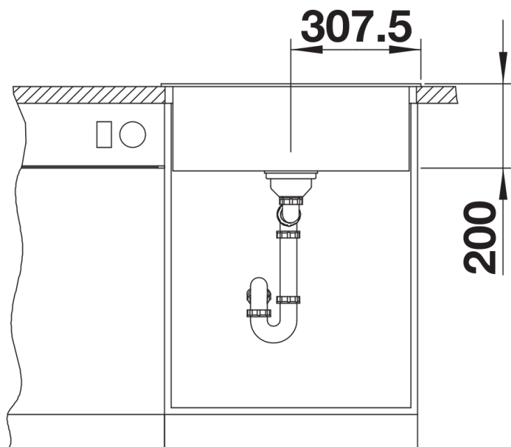
Vooraanzicht
