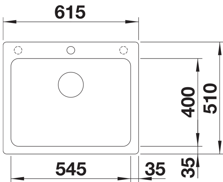
Bovenaanzicht
