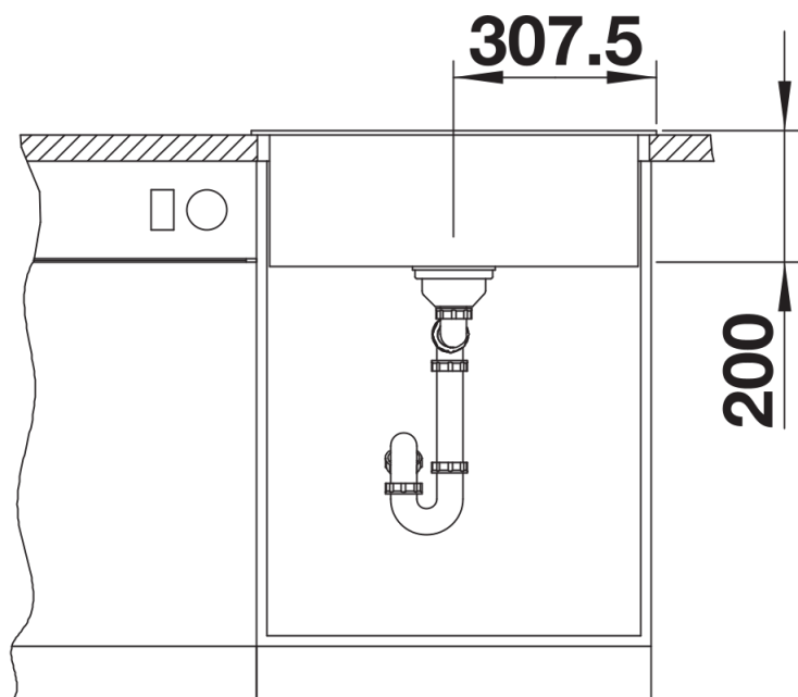
Vooraanzicht
