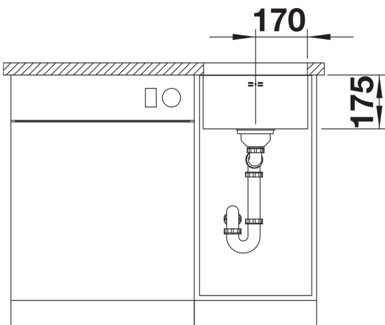
Vooraanzicht
