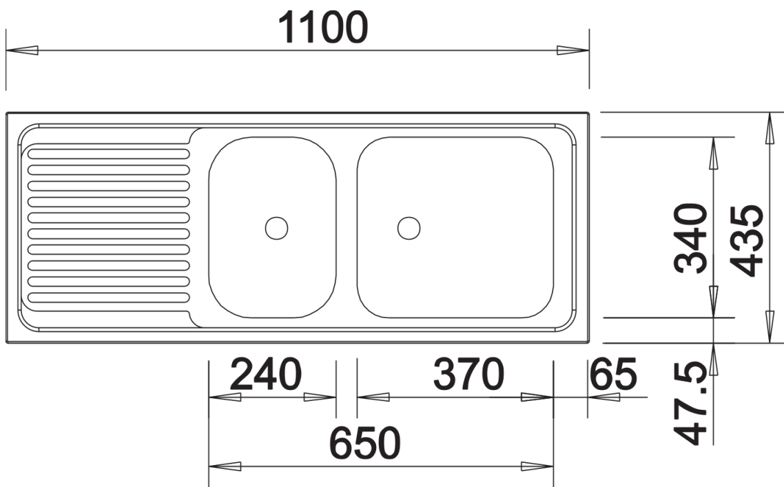
Bovenaanzicht
