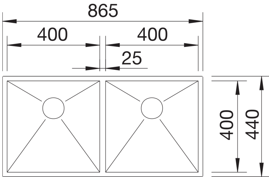
Bovenaanzicht
