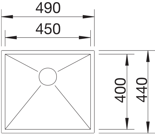
Bovenaanzicht
