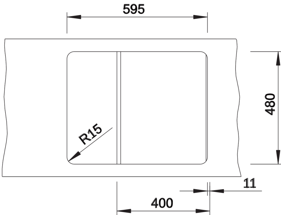
Uitgesneden
