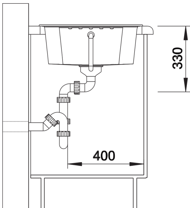
Zijaanzicht
