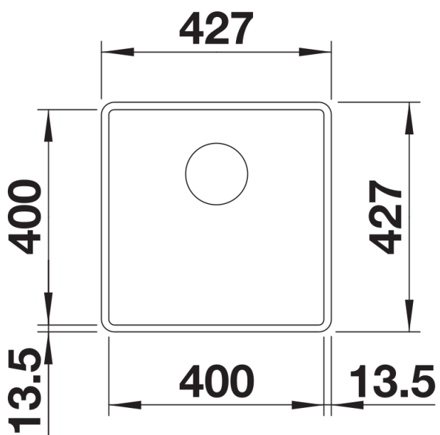
Bovenaanzicht
