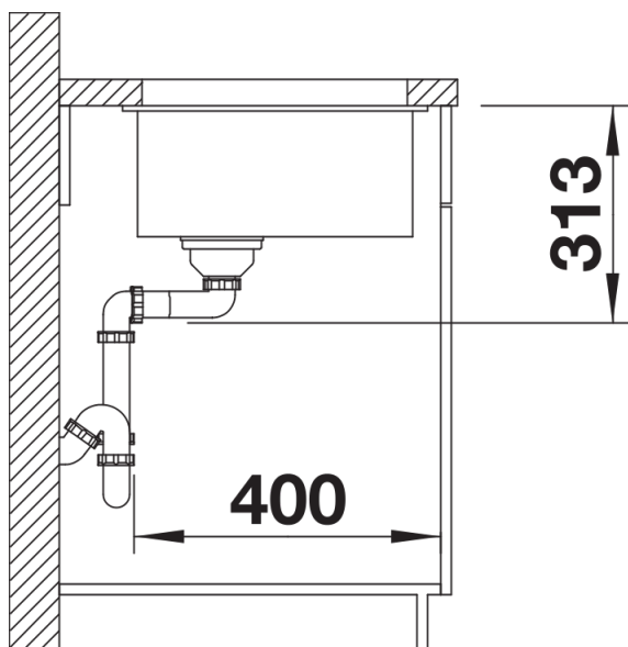
Zijaanzicht
