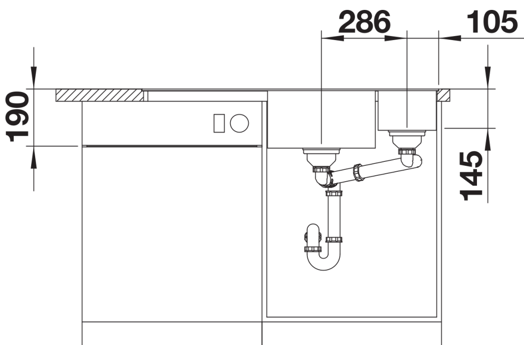
Vooraanzicht
