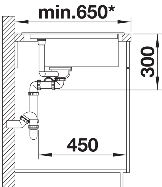
Zijaanzicht
