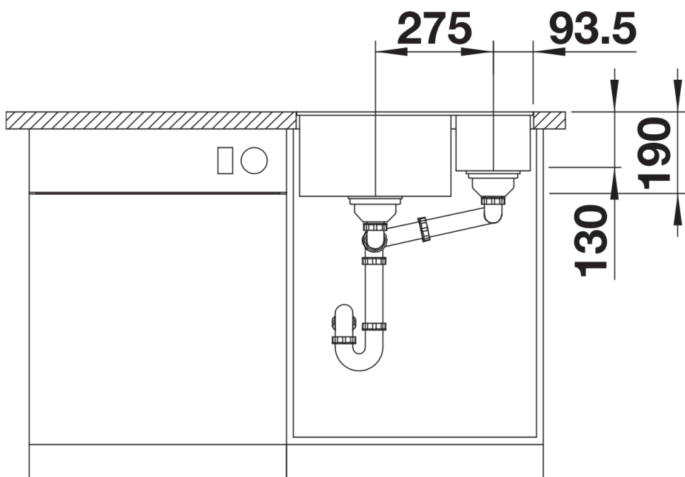
Vooraanzicht
