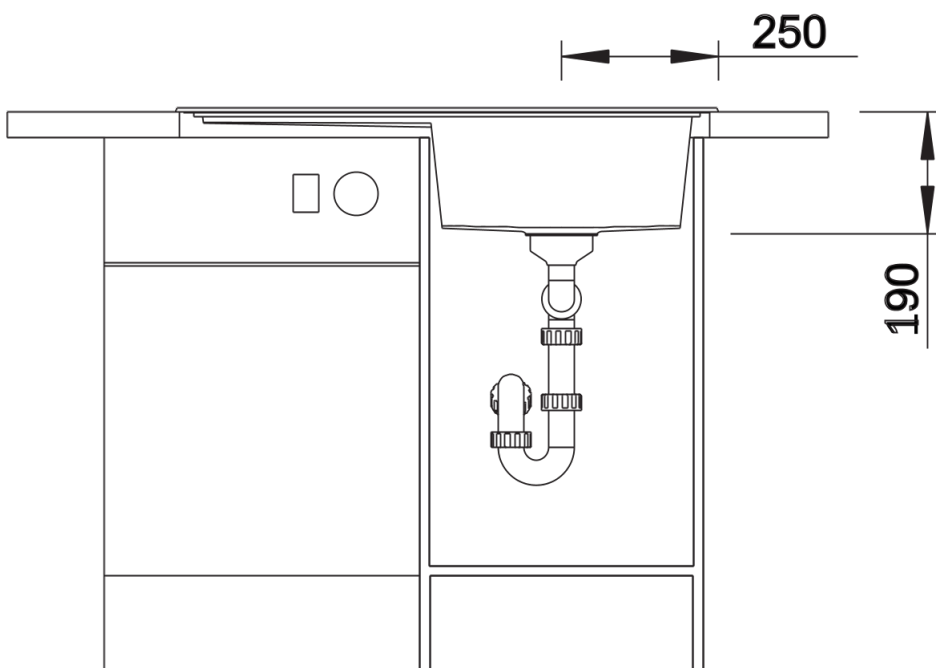
Vooraanzicht
