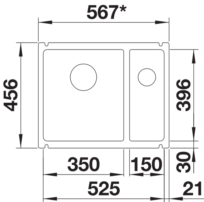
Bovenaanzicht
