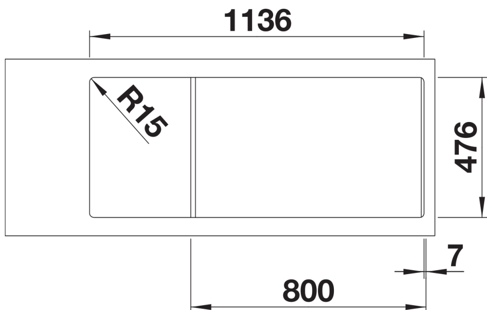
Wycięcie
