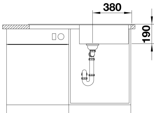
Вид спереди
