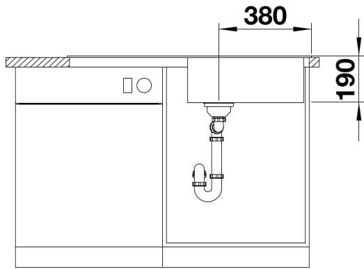
Вид спереди
