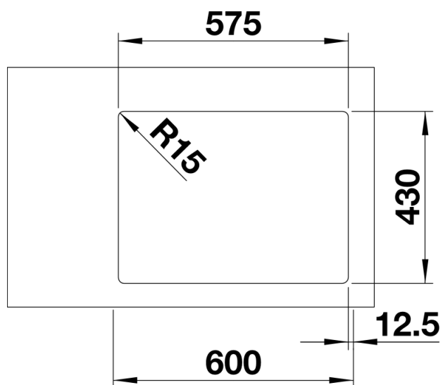
Вырез
