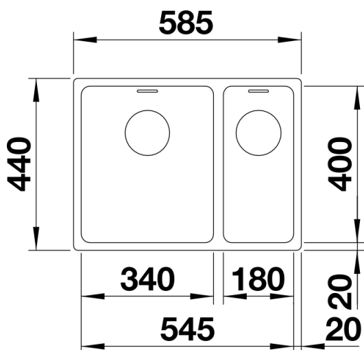
Вид сверху
