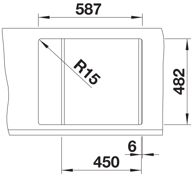
Вырез
