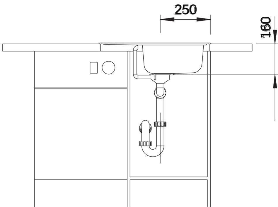
Вид спереди
