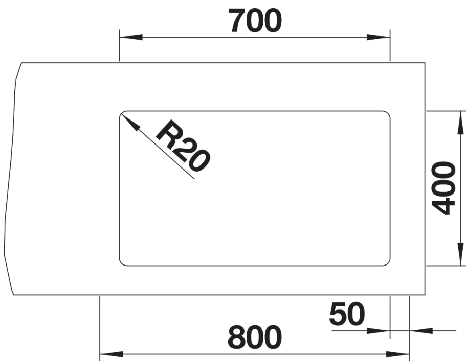
Виріз
