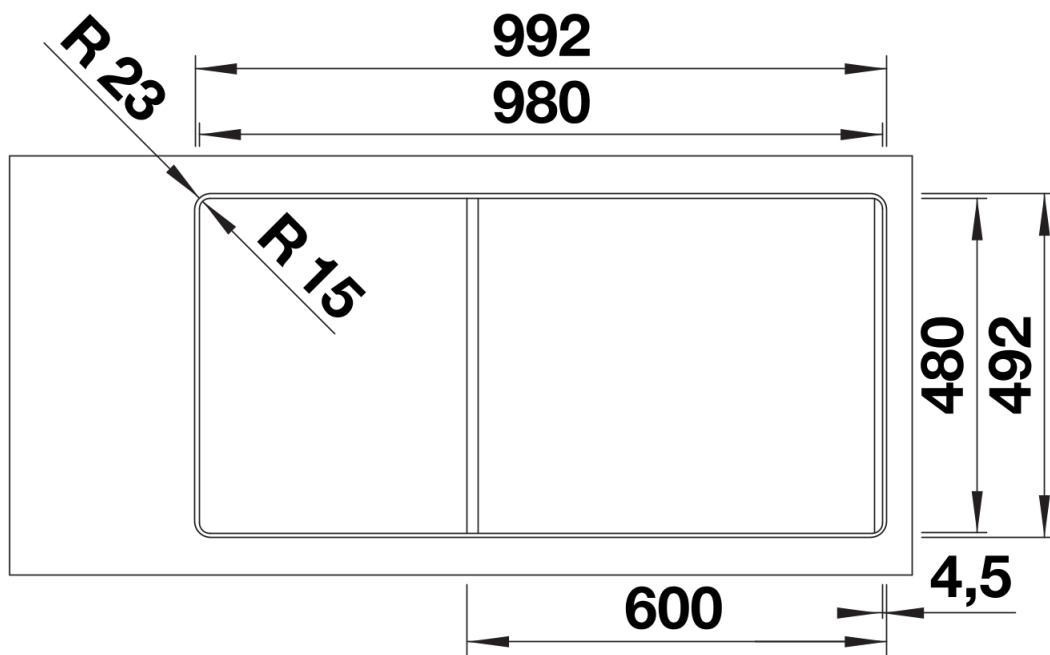
Виріз
