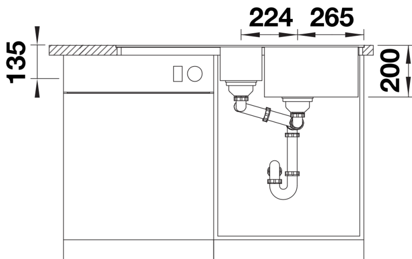
Фронтальний вигляд
