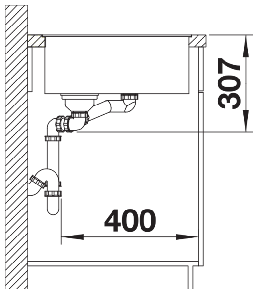
Боковий вигляд
