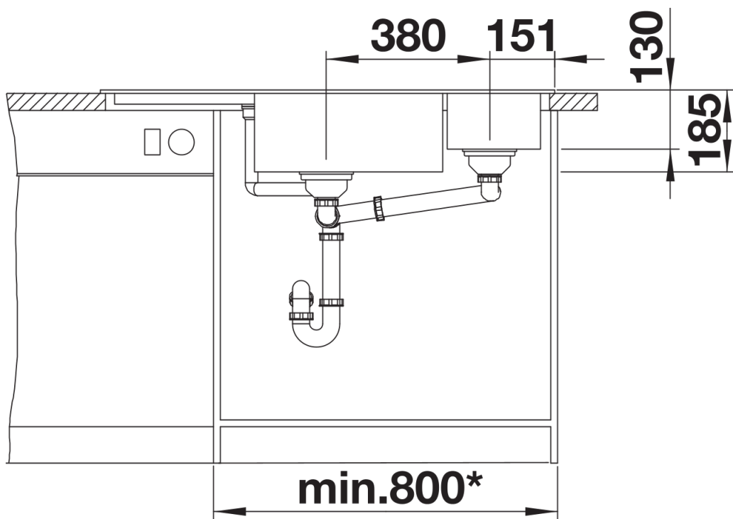
Фронтальний вигляд
