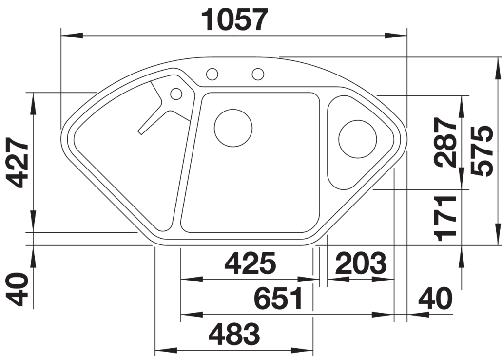
Вигляд зверху
