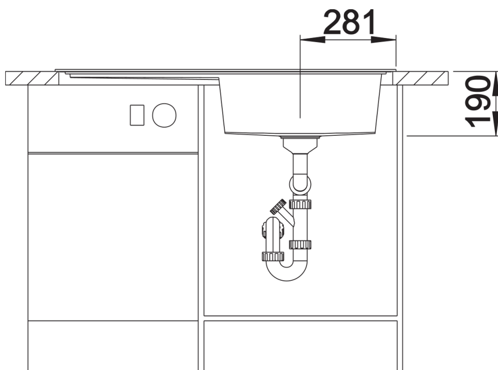
Фронтальний вигляд
