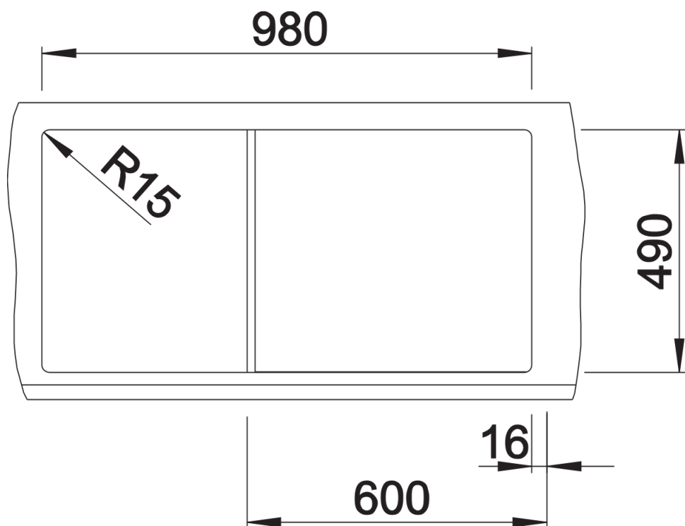
Виріз
