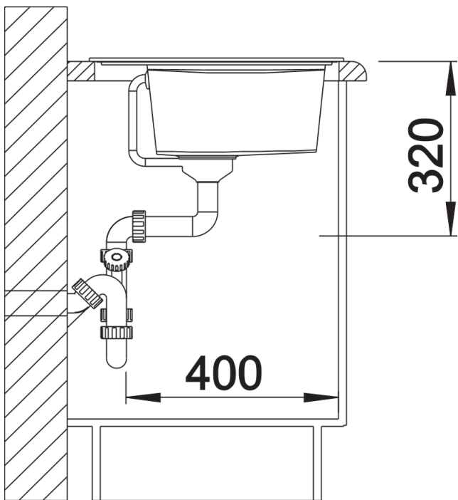
Боковий вигляд
