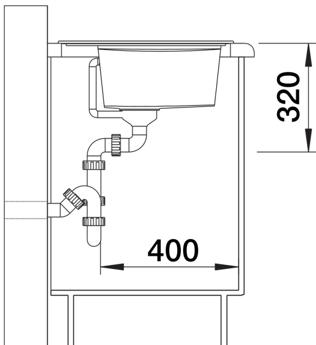
Боковий вигляд
