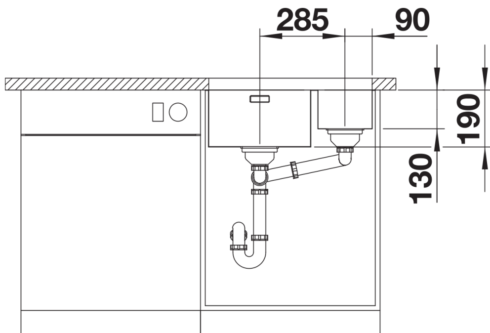
Mặt cắt trước
