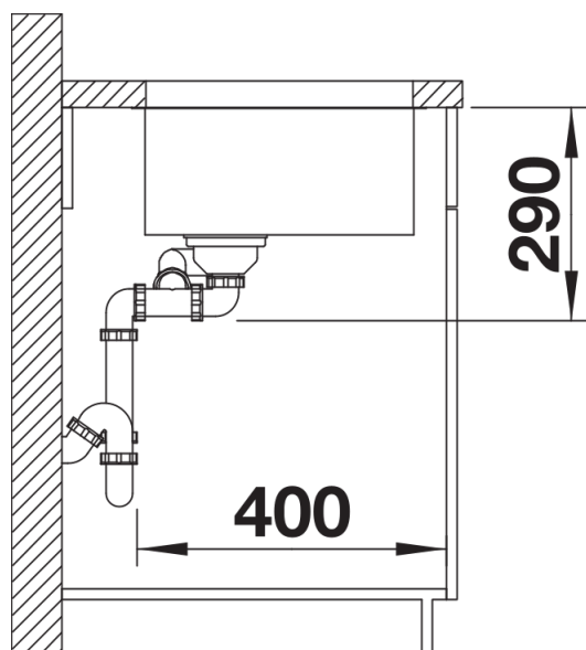
Mặt cắt bên
