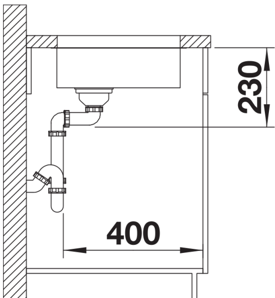
Mặt cắt bên
