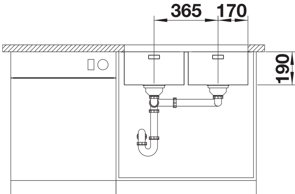
Mặt cắt trước
