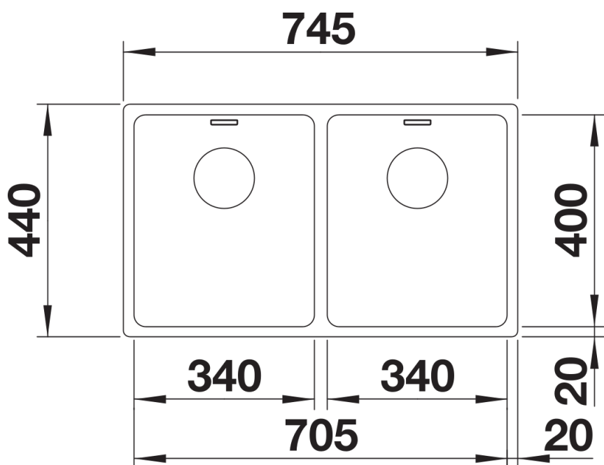
Mặt cắt trên
