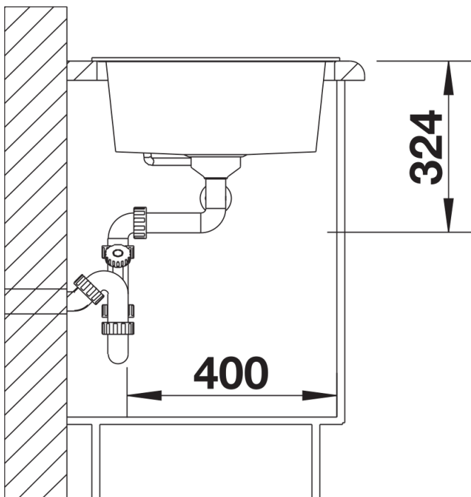
Mặt cắt bên
