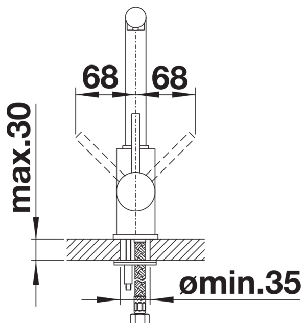
Mặt cắt bên tay cầm 2D
