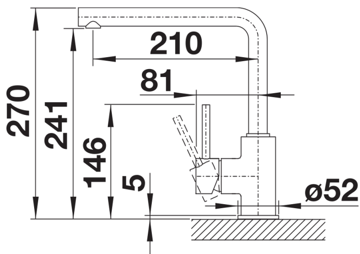
Mặt cắt bên
